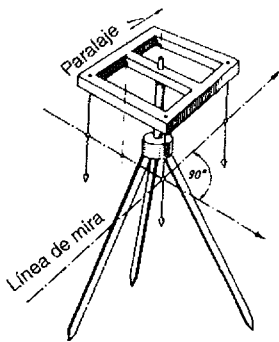
LÁMINA 23. Una groma. La groma permite hacer jalonomientos en ángulos de 90°. Modelo conservado en la Saalburg. Dibujado por F. Kretschmer, La technique romaine, 1966.
