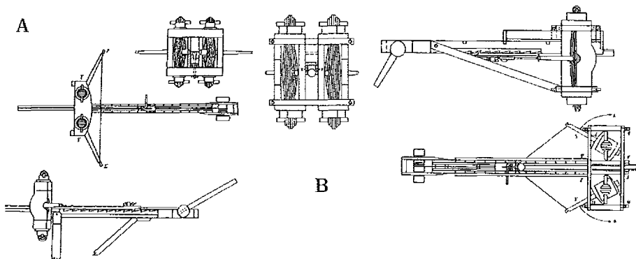
LÁMINA 27. La artillería. A. Esta máquina sirve para arrojar flechas. Dibujo superior: vista desde lo alto. Dibujo del medio: vista en plano. Dibujo inferior: vista lateral. Según E. W. Marsden, Greek and Roman Artillery , 1971; B. Esta máquina sirve para arrojar piedras. Dibujo superior izquierda: planta. Dibujo inferior izquierda: vista lateral. Dibujo a la derecha: vista de frente. Según E. W. Marsden, Greek and Roman Artillery , 1971.
