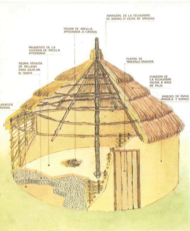
Esquema de una vivienda castreña
