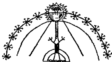
Diagrama que representa un eclipse de sol
