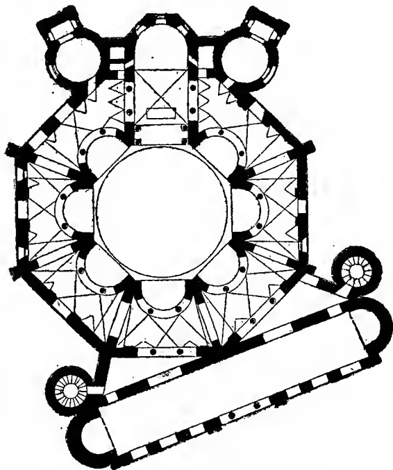
FIG. 28. Plan of St. Vitale, Ravenna.
