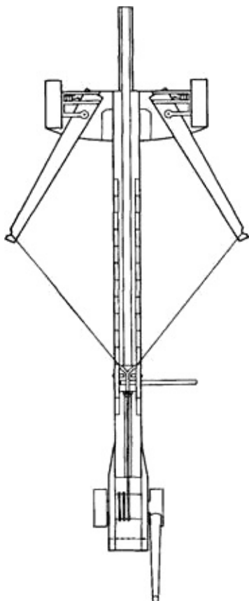
Catapulta con resorte de bronce de Ctesibio. (Según Mardsen, Greek and Roman Artillery Technical Treatises , p. 174, diagrama 9; reproducido con permiso de Oxford University Press)
