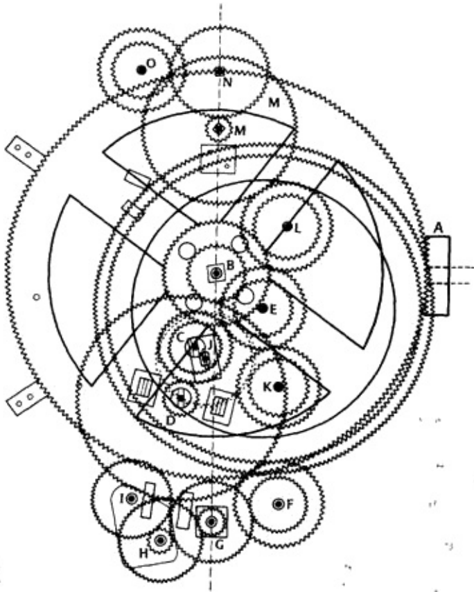
El engranaje de Anticitera (Según el dibujo de B. Pope en Price, Gears , p. 37, fig. 29, reproducida con autorización de la American Philosophical Society .)
