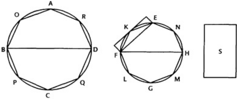
Demostración de Euclides por el método de la exhaución. (Basada en Thomas, Greek Mathematical Works , i. 461)
